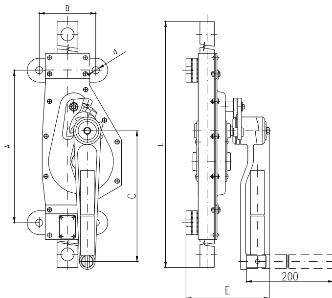
Obr.1 Zdvihák typ 15-00 CON - W
