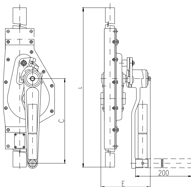
Obr.2 Zdvihák typ 15-00 CON
