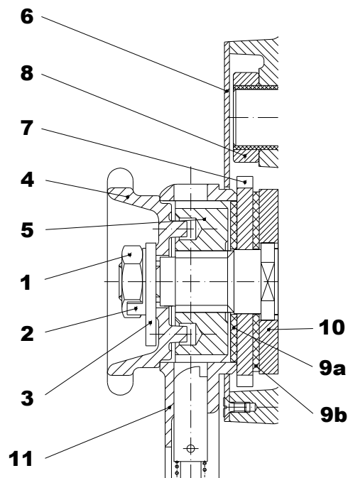
Obr. 11.3 - Montáž brzdy
