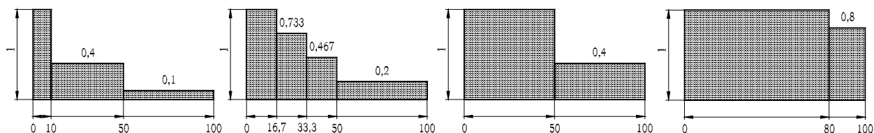
1. диаграмма нагрузки
