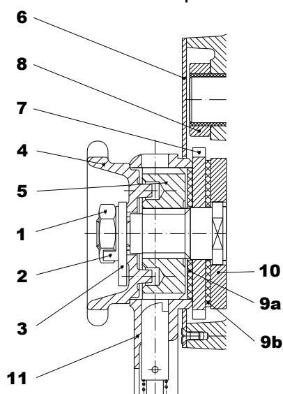
Рис. 11.4. Регулировка тормоза
