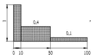
Zátěžový diagram 1
