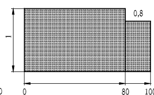
Zátěžový diagram 4
